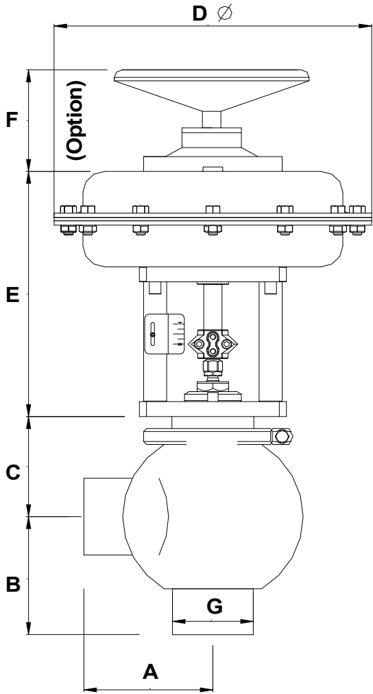
FLANGIA FLANGE
